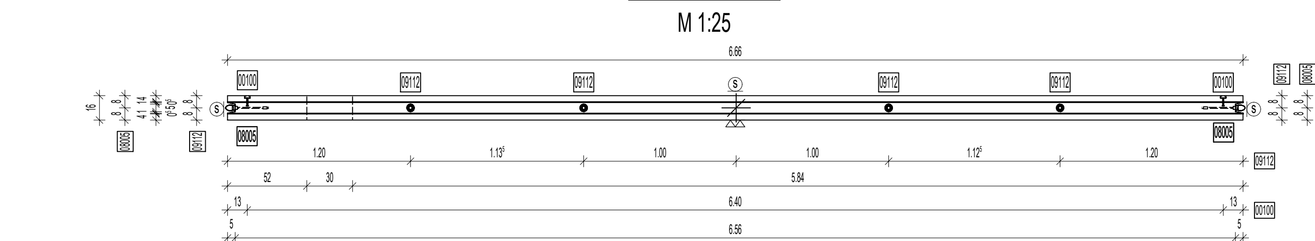
Draufsicht 1-1 M 1:25
