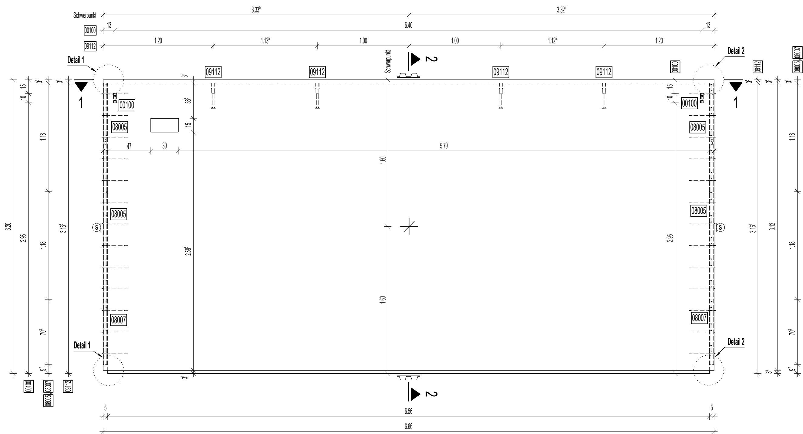
Draufsicht 1-1 M 1:25
