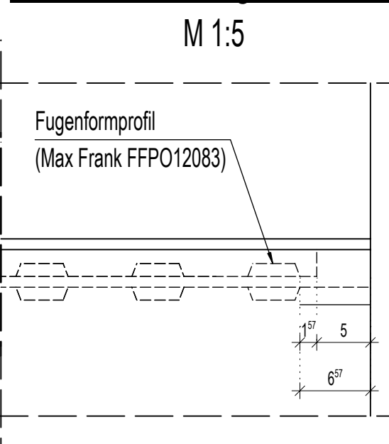
Ansicht Stoßfuge - Detail 2 M 1:5
