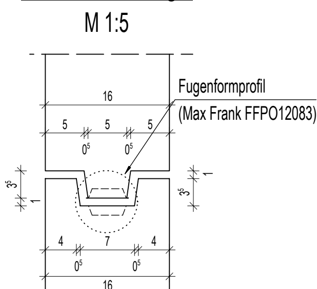
Detail Stoßfuge M 1:5
