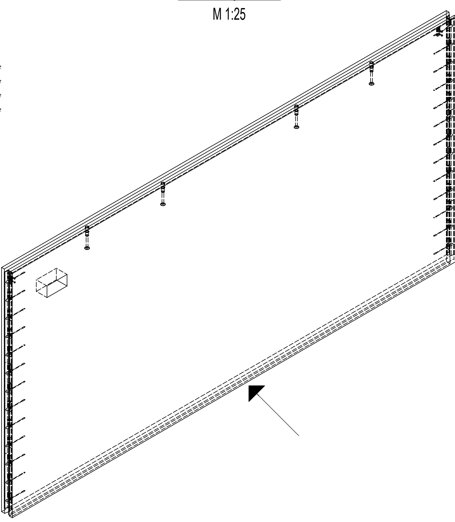
3D Perspektive M 1:25
