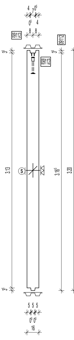
Schnitt 2-2 M 1:25
