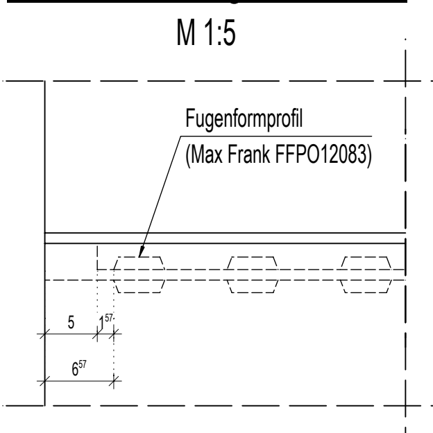
Ansicht Stoßfuge - Detail 1 M 1:5
